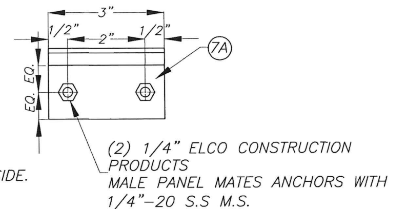
DETAIL X ELEVATION SCALE= N.T.S.
