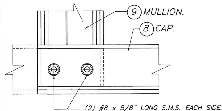
DETAIL 1 SCALE= N.T.S.
