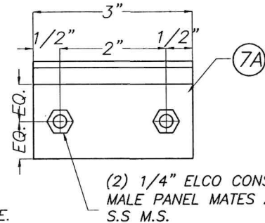
DETAIL X ELEVATION SCALE= N.T.S.
